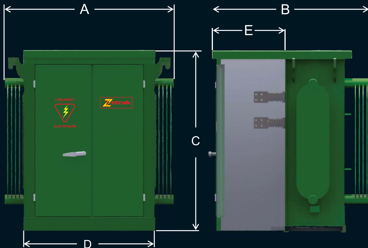
DIMENSIONES Y PESOS APROXIMADOS OPERACIÓN RADIAL Y ANILLO EN ALUMINIO
